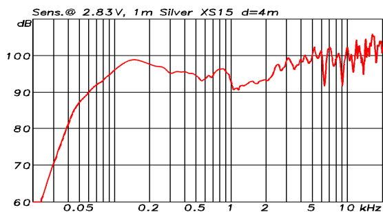
XS 15 Réponse en fréquence
