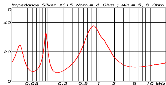
XS 15 courbe d'impédance
